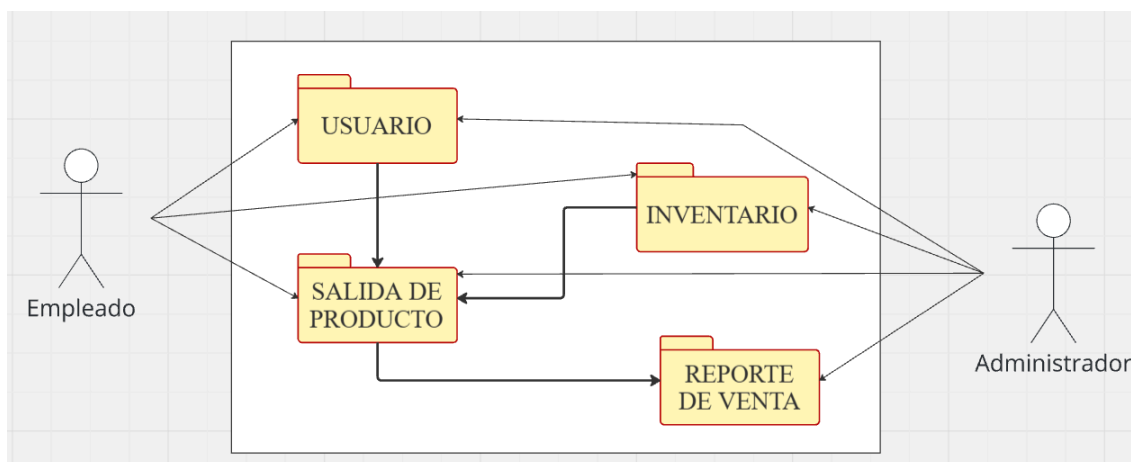
Figura 01. Diagrama de paquetes.
