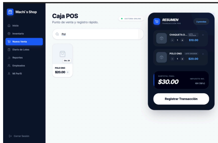
Interfaz Gráfica Vista Escritorio
